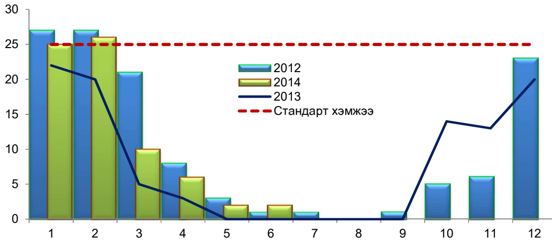
Зураг 24. Хүхэрлэг хийн агууламж, сараар, мг/м 3
